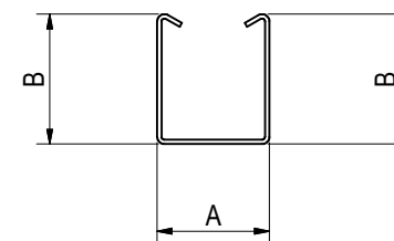
Kształtownik U13 [mm]
